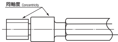
同軸度検査用ねじプラグゲージ Thread plug gauge for concentricity
