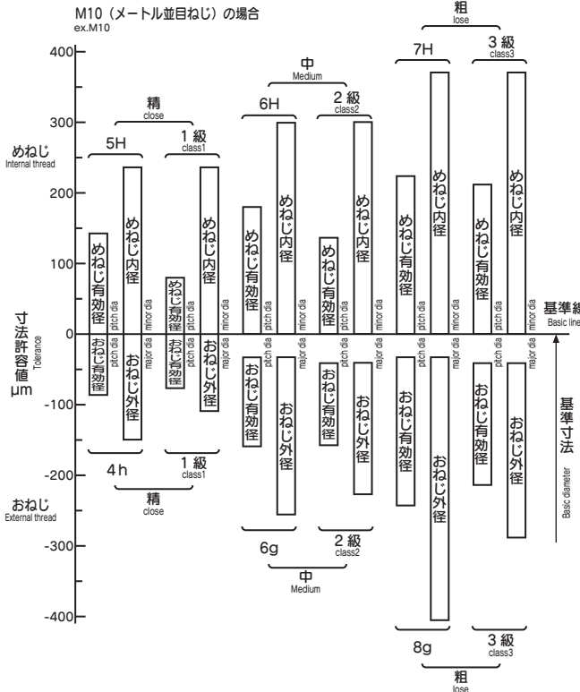
製品ねじ ISO 等級と 1,2,3 等級の公差位置
